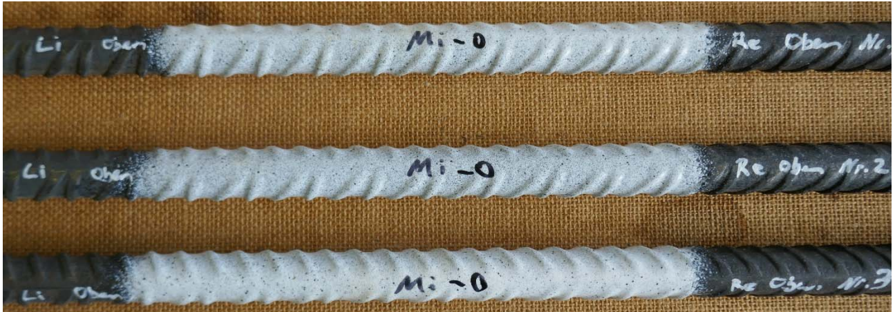
Abbildung 5: Ansicht der Anker im Bereich der Beschichtung vor der Korrosionsprüfung.
